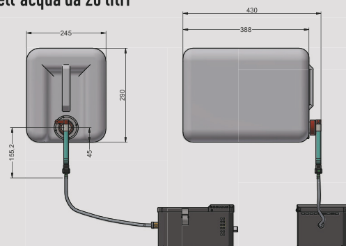
Serbatoio dell'acqua da 20 litri
